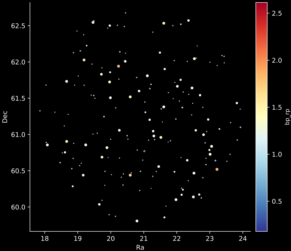
APOGEE DR17 Field: [CVZTILE_091+24_btx] Stars: 170
