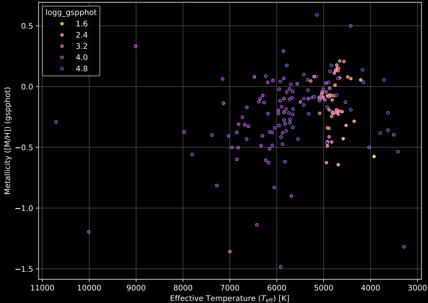
APOGEE DR17 Field: [CVZTILE_091+24_btx] Stellar Population Parameters (n= 170)
